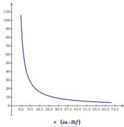
omega(tau) (1/s)
