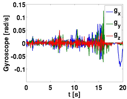
(d) Gyroscope data with fans at full
