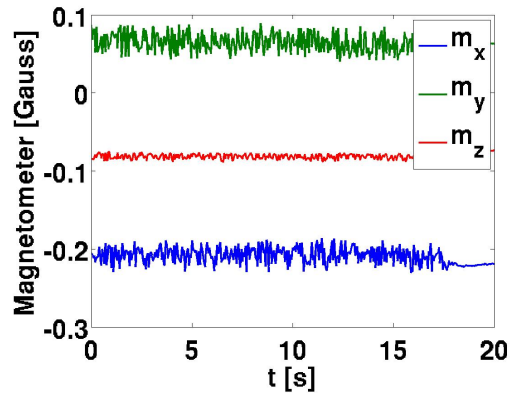
(d) Magnetometer data with fans at full
